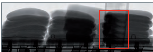
На рентгеновском изображении, полученном системами Eagle, выявляются запрещенные предметы в грузах высокой плотности.
